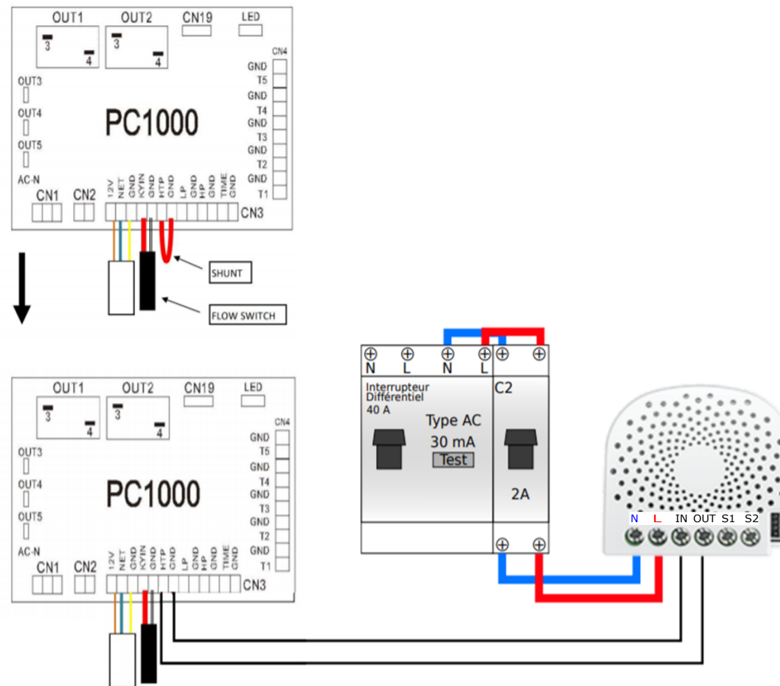
Schéma de câblage pour commander une Prima en Marche-arrêt:
